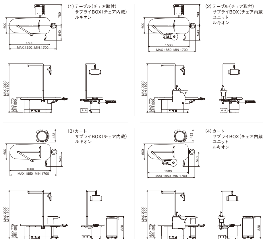
標準4パターン 寸法図(1/80)
