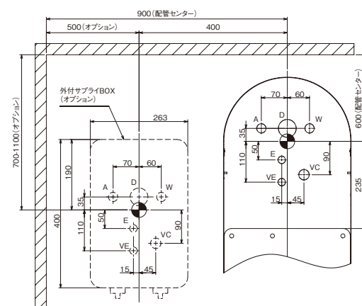
立ち上がり配管図(1/20)
