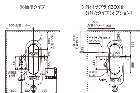
配置図(1/80)
